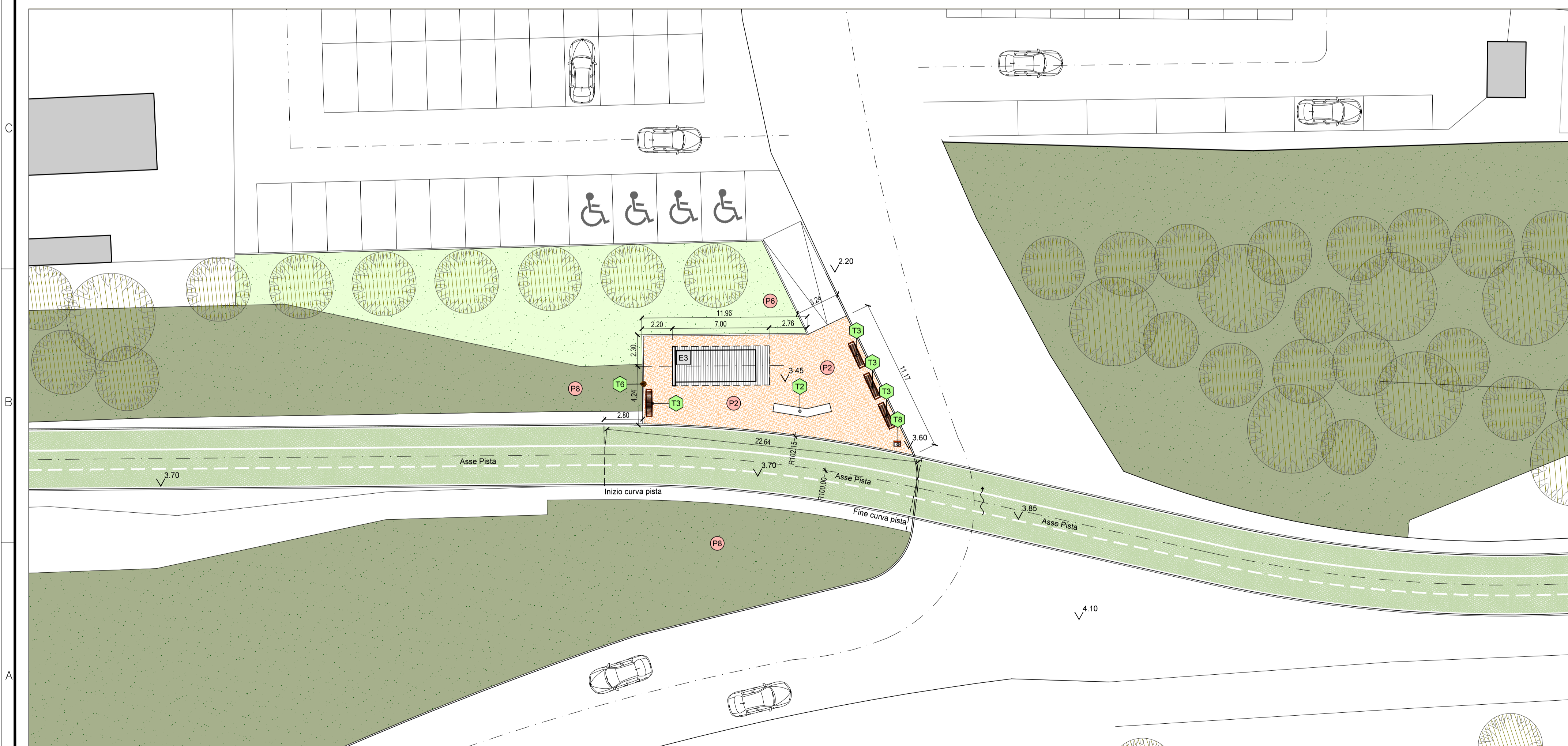
ACCESSO 9 PORTO TURISTICO - PROGETTO: PLANIMETRIA - SCALA 1:200
