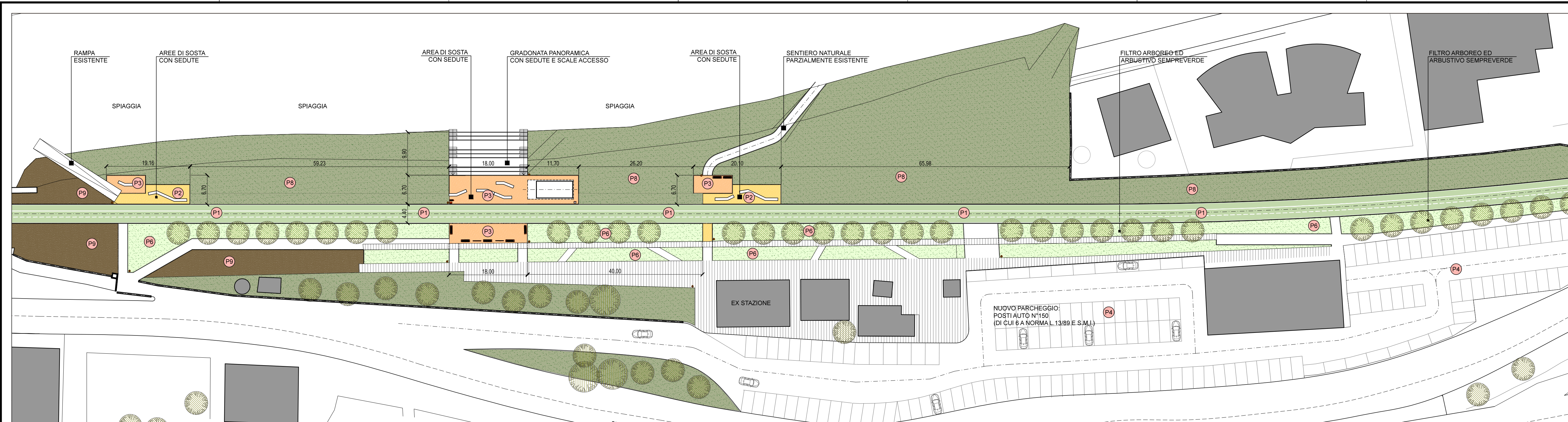
ACCESSO 7 EX STAZIONE DI FOSSACESIA - PROGETTO: INQUADRAMENTO - SCALA 1:500
