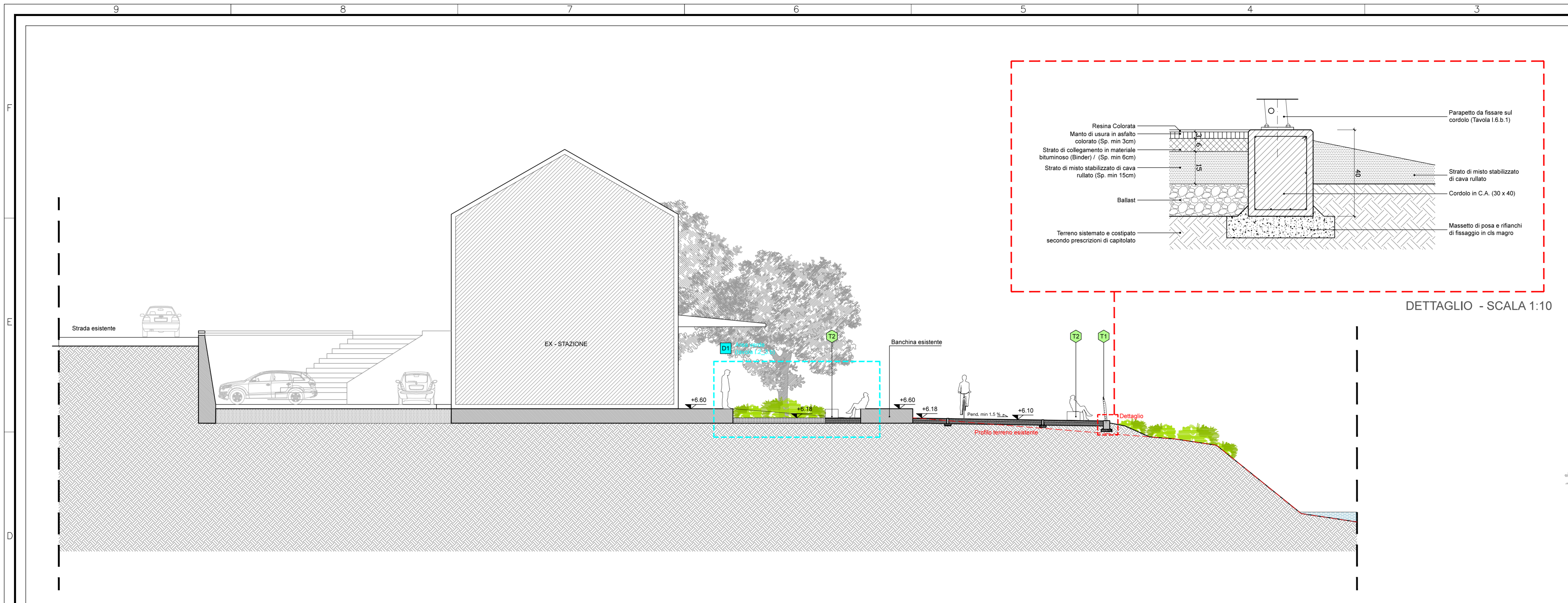
ACCESSO 3 SAN VITO CHIETINO - PROGETTO: SEZIONE A - A - SCALA 1:100
