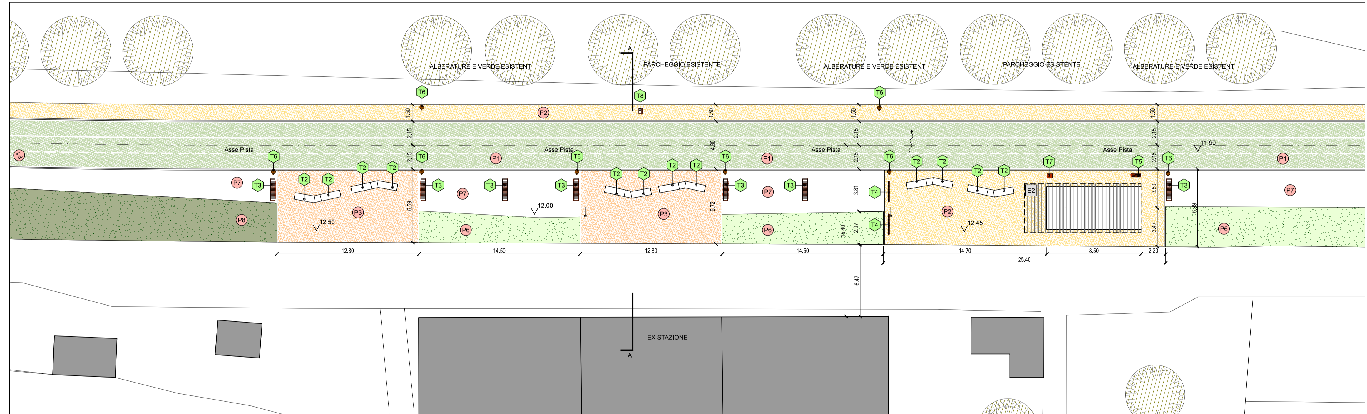
ACCESSO 13 EX STAZIONE VASTO - PROGETTO: PLANIMETRIA - SCALA 1:200
