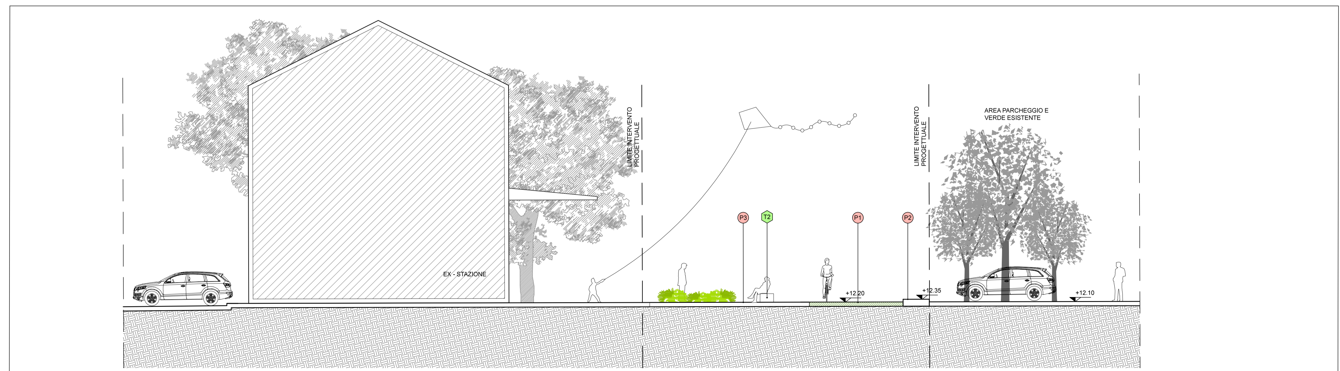
ACCESSO 13 EX STAZIONE VASTO - PROGETTO: SEZIONE A - A _ SCALA 1:100
